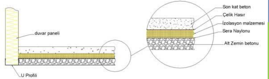
İnşai Tip Zemin / Duvar Paneli Birleşim Detayı
